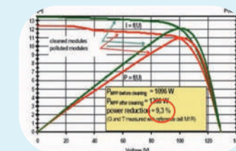
汚染による太陽光発電出力低下最大 9.3%
