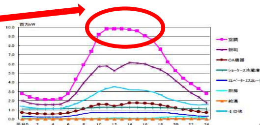
【時間帯別電力需要(機器別)】
